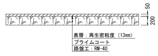
アスファルト舗装構成図 (車道部B) S = 1 : 50
