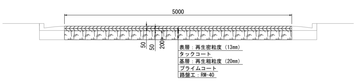
アスファルト舗装構成図 (車道部A) S = 1 : 50
