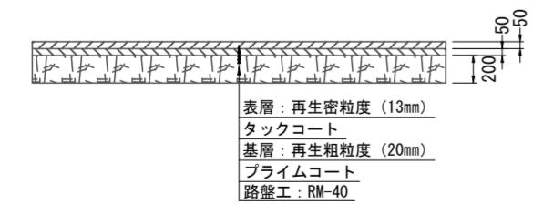
アスファルト舗装構成図 (車道部A) S = 1 : 50
