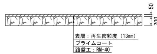
アスファルト舗装構成図 (車道部) S = 1 : 50
