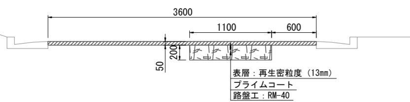
横断図No.5 S = 1 : 50
