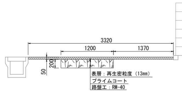
アスファルト舗装構成図 (車道部B) S = 1:50
