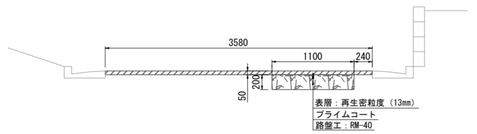
アスファルト舗装構成図 (車道部B) S = 1 : 50
