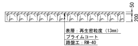
アスファルト舗装構成図 (車道部B) S = 1:50
