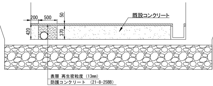
架道橋下横断図(詳細) S = 1:50
