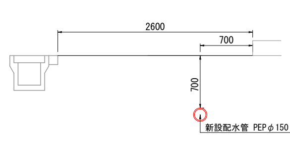
No.20(市道車道部)
