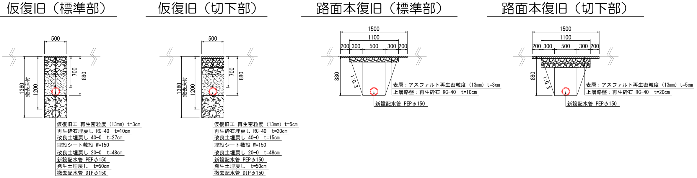
県道歩道部管撤去同時施工標準横断面図 S = 1 : 50
