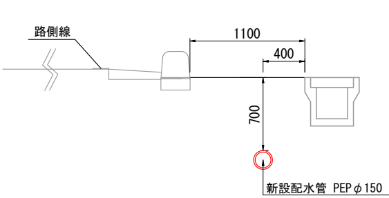
NO.3(県道歩道標準部)
