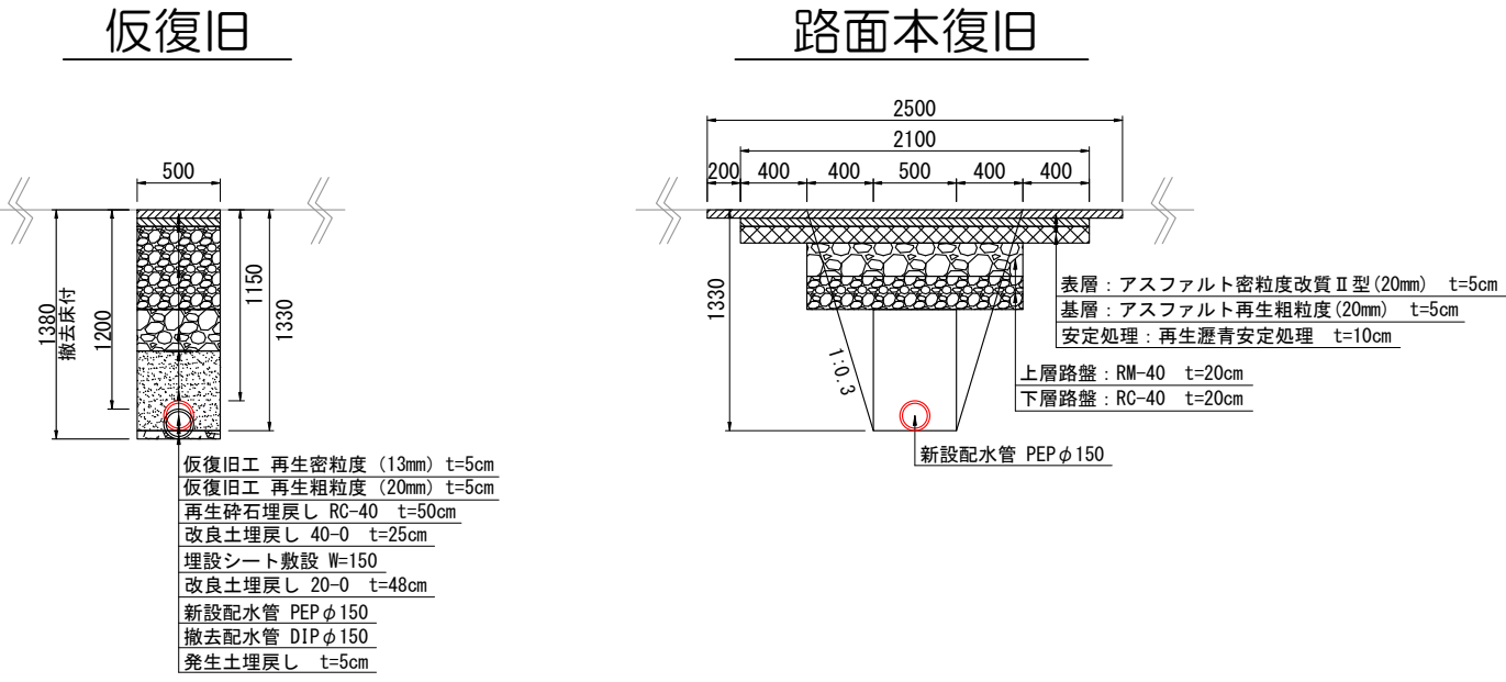
県道車道部管撤去同時施工標準横断面図 S = 1 : 50
