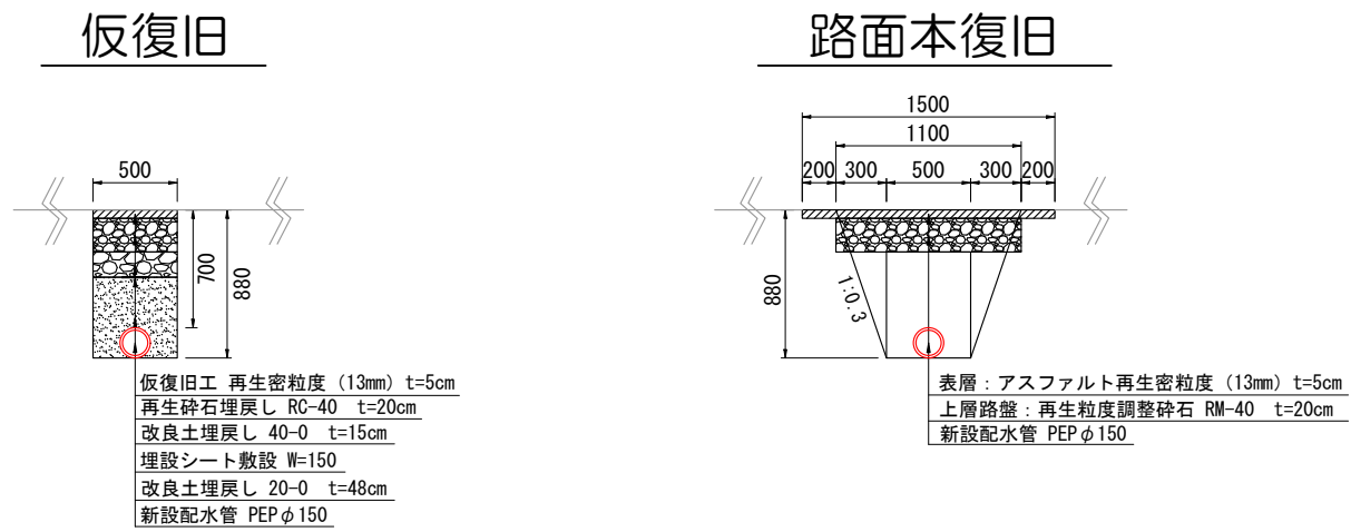
市道車道部標準横断面図 S = 1 : 50
