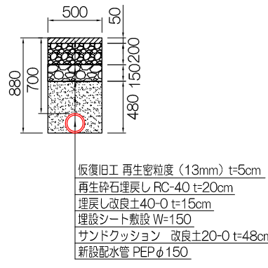
仮復旧（歩道）
