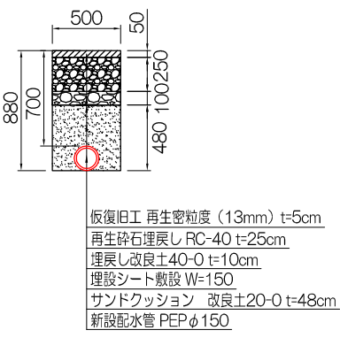
仮復旧（車道）
