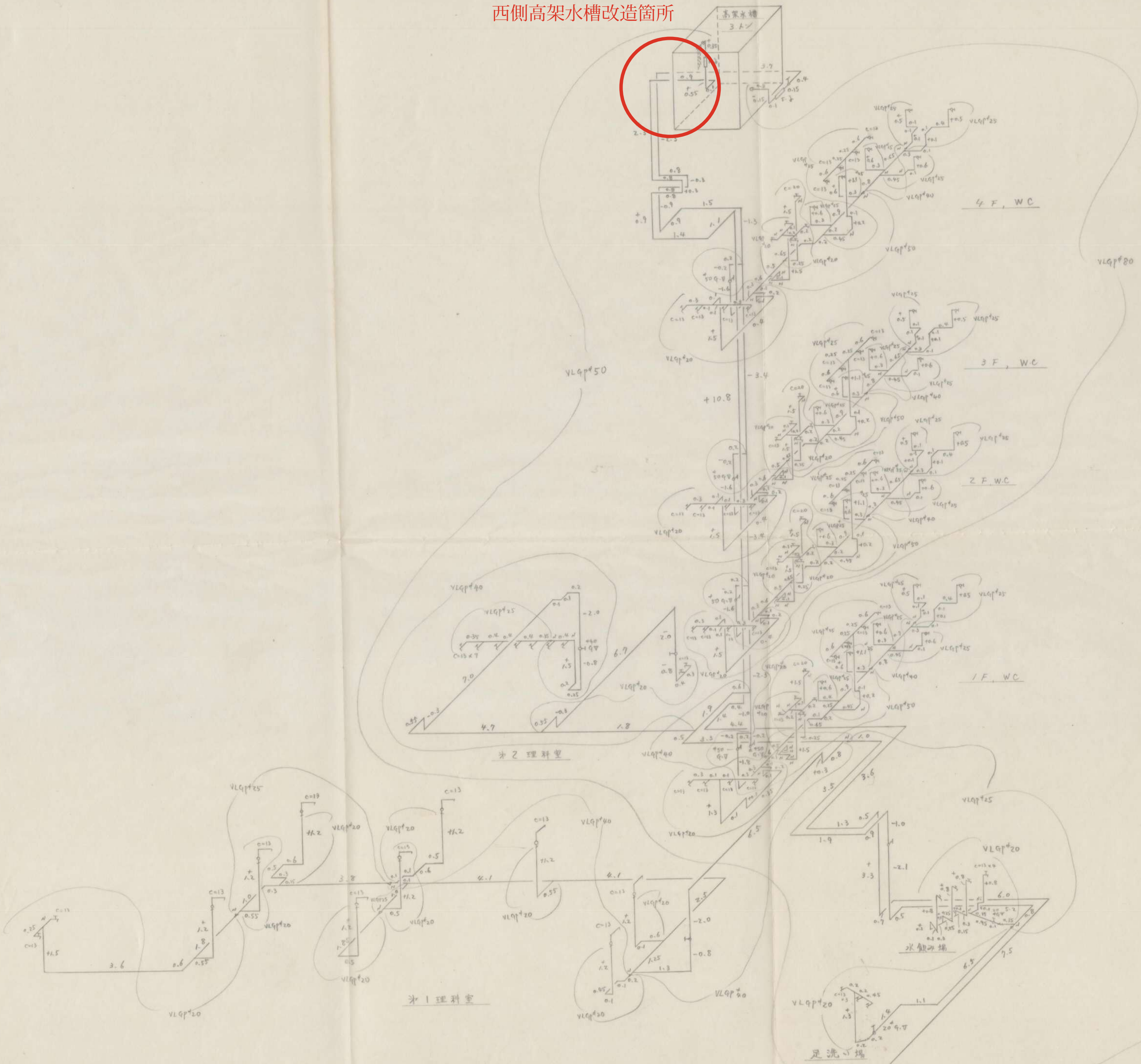
三浦市立初等小学校増築工事 高架水槽以下給水管立面図(40II)
