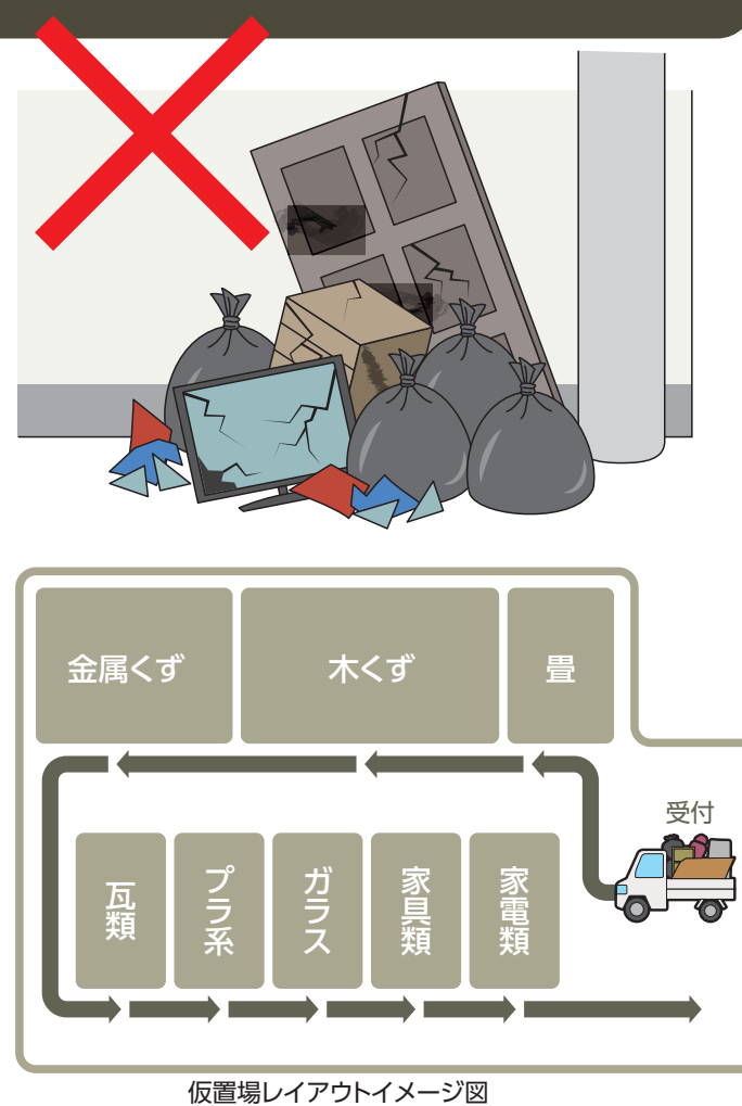
仮置場レイアウトイメージ図
