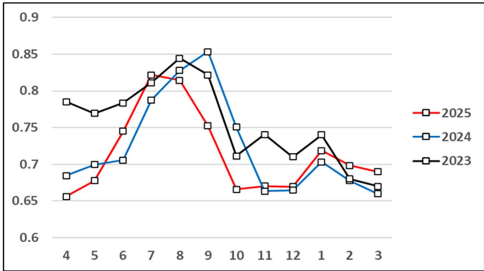
図7 東部浄化センターの使用電力量及び電力原単位 iii
