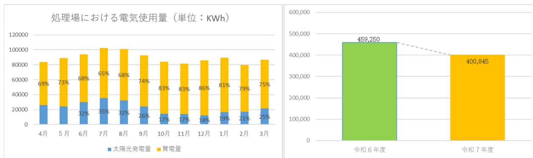
図5 太陽光発電量の割合
